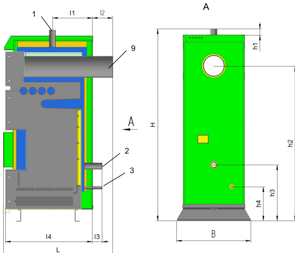
Рисунок 1 - Габаритные и присоединительные размеры Котлов моделей L-12+102
