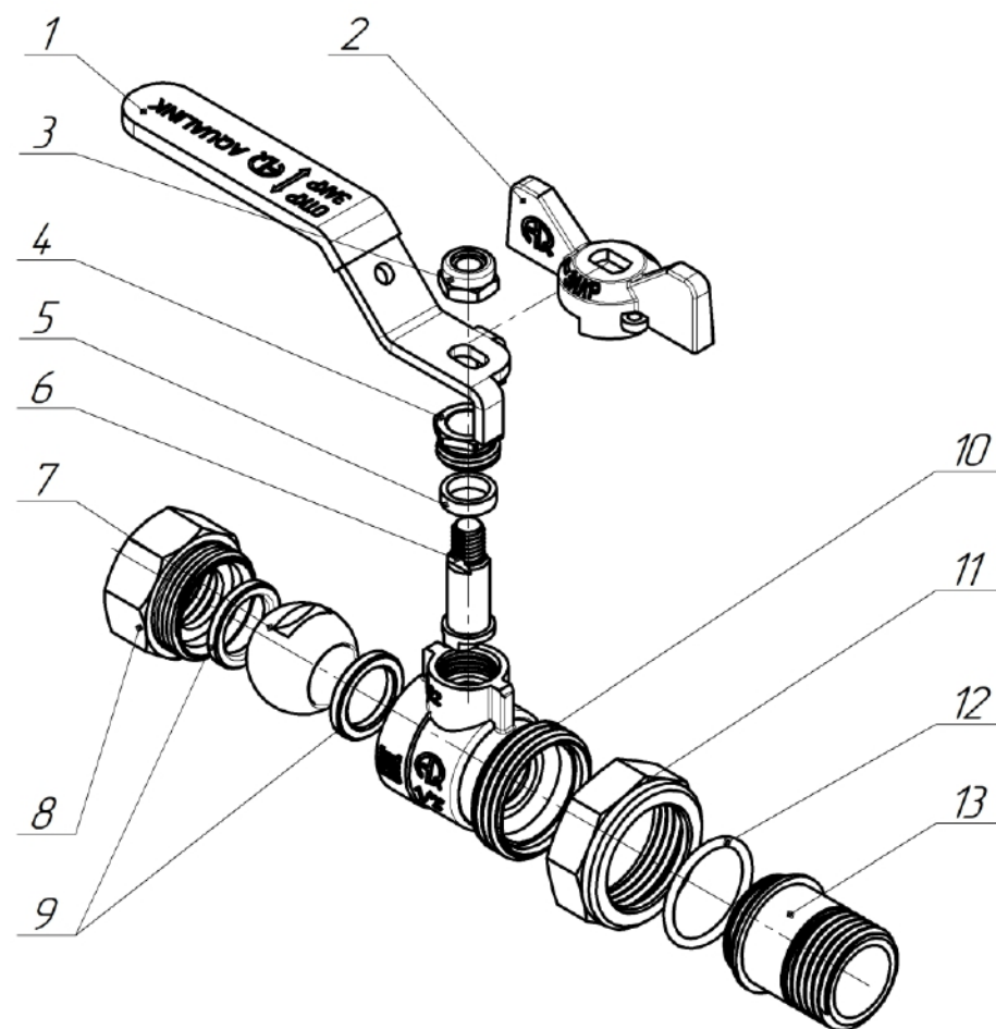
Рисунок 2 – Общий вид и конструкция изделия
