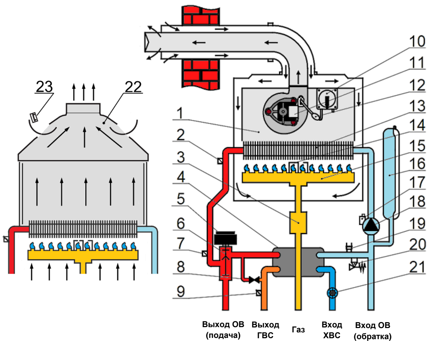
Рис. 2 Функциональная схема котлов серии Arderia D и Arderia D Atmo (слева)
